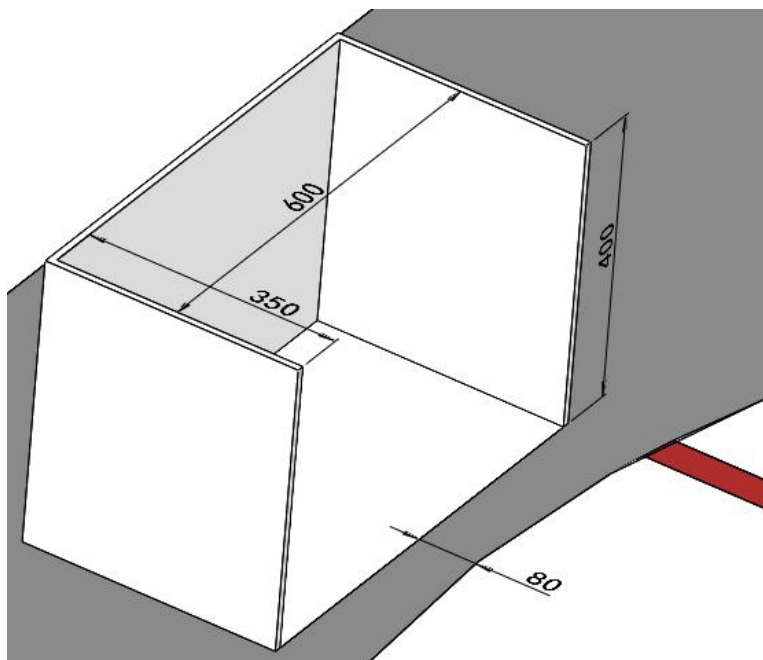
图 7 住户 1 标识尺寸（单位：mm）
